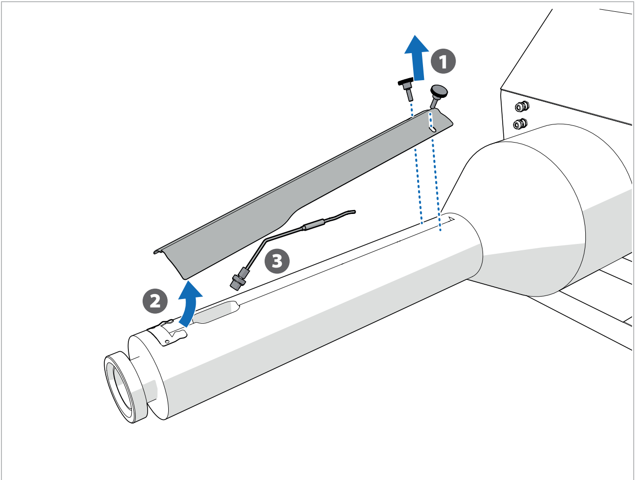
Abbildung 11 Sensor ausbauen
